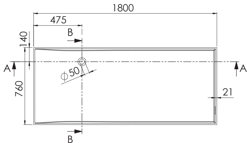
SCHNITT A-A
