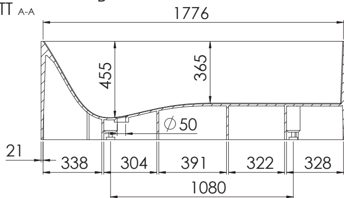
SCHNITT B-B
