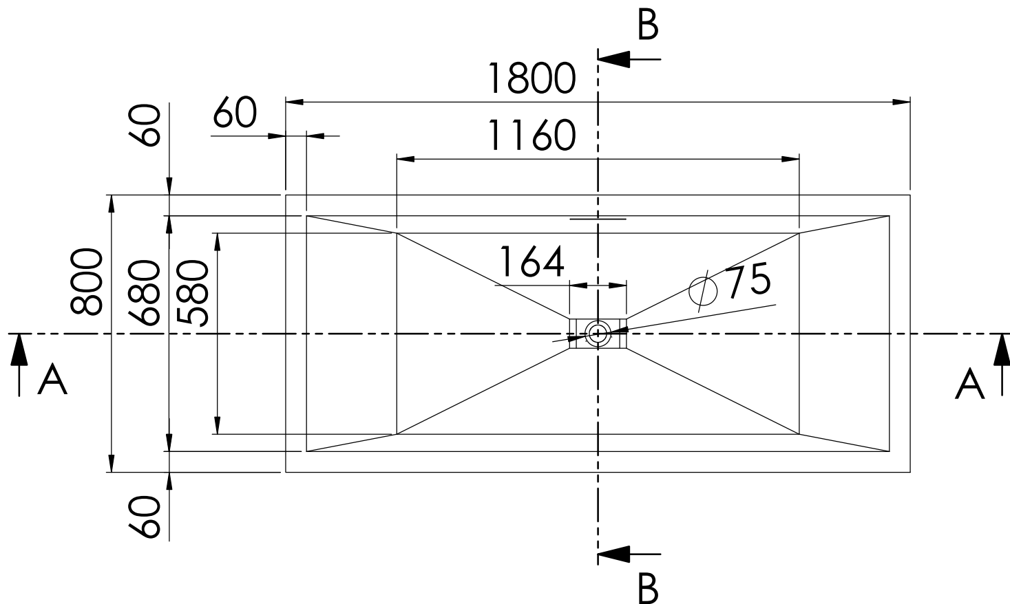
SCHNITT A-A
