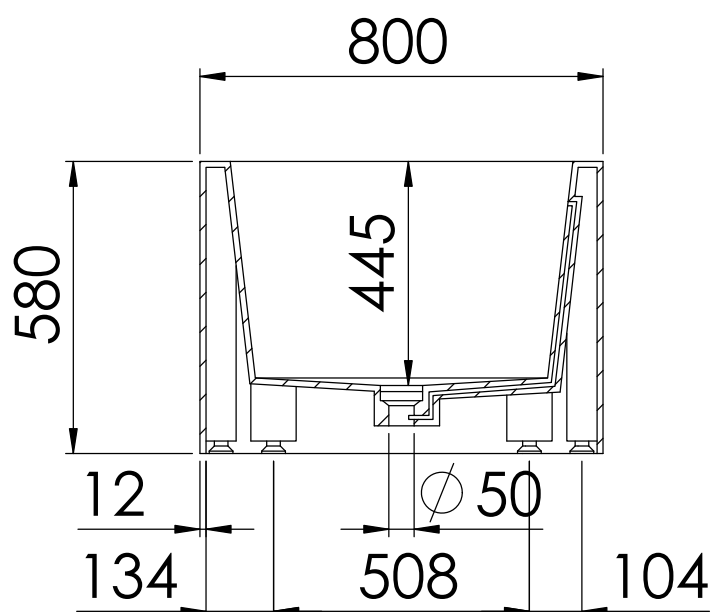
SCHNITT B-B
